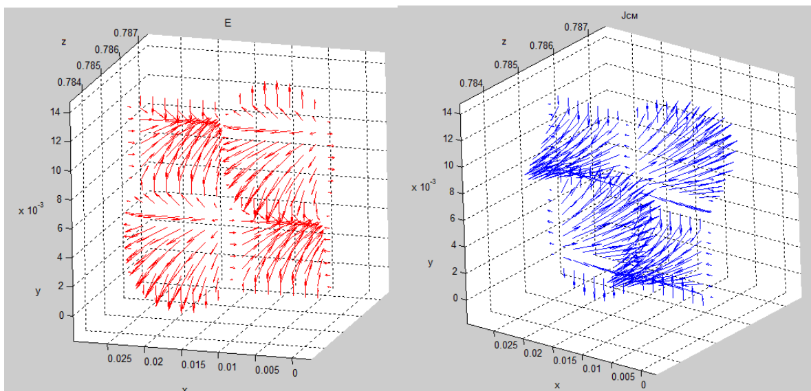
Электрическое поле.
