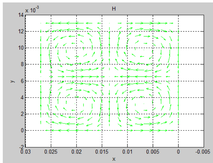
Магнитное поле
