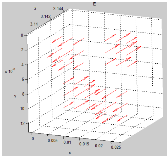
Электрическое поле.
