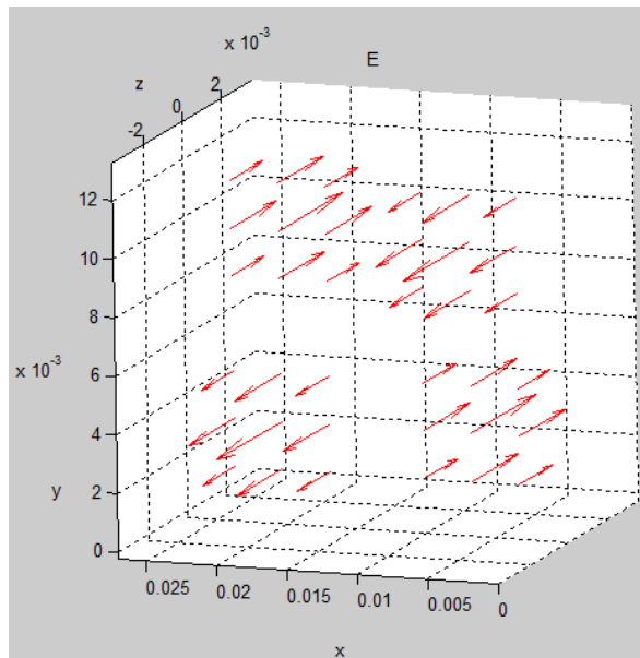
Электрическое поле.
