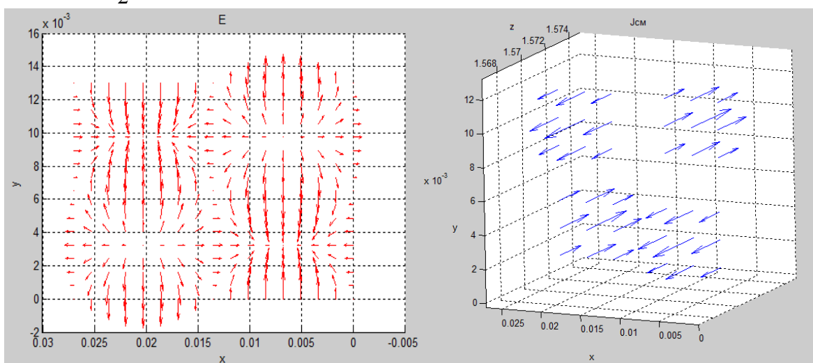
Электрическое поле.
