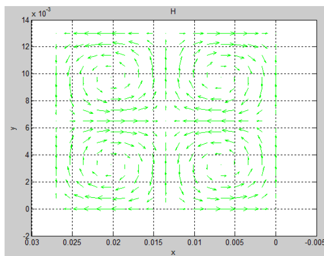
Магнитное поле
