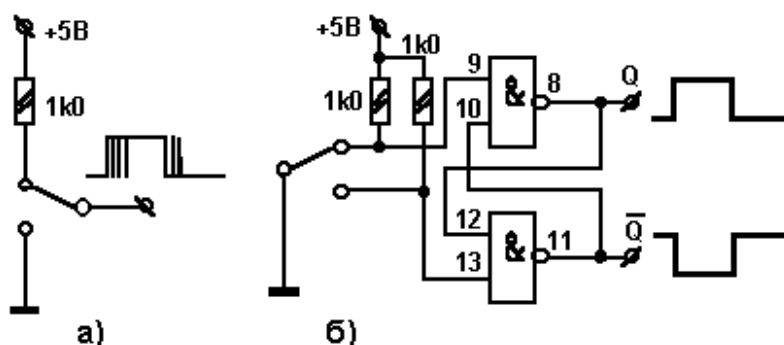
Рис. 11. Подавление дребезга механических контактов с помощью RS-триггера
