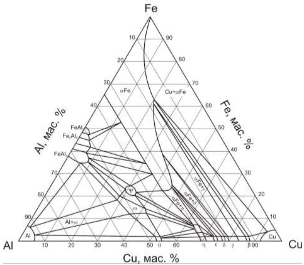
Рисунок 1.9 – Изотермический разрез диаграммы состояния Fe-Cu-Al при 600 °C [134].
