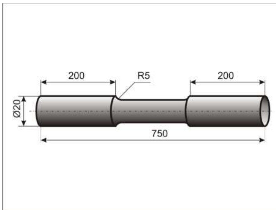
Рисунок 2.3 – Схема образца для проведения испытаний в условиях одноосного статического растяжения
