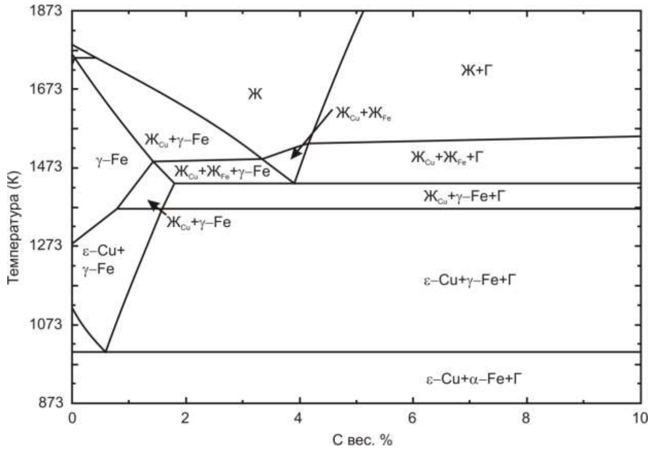
Рисунок 1.5 - Разрез диаграммы Fe-Cu-C при 5 мас. % меди [131]
