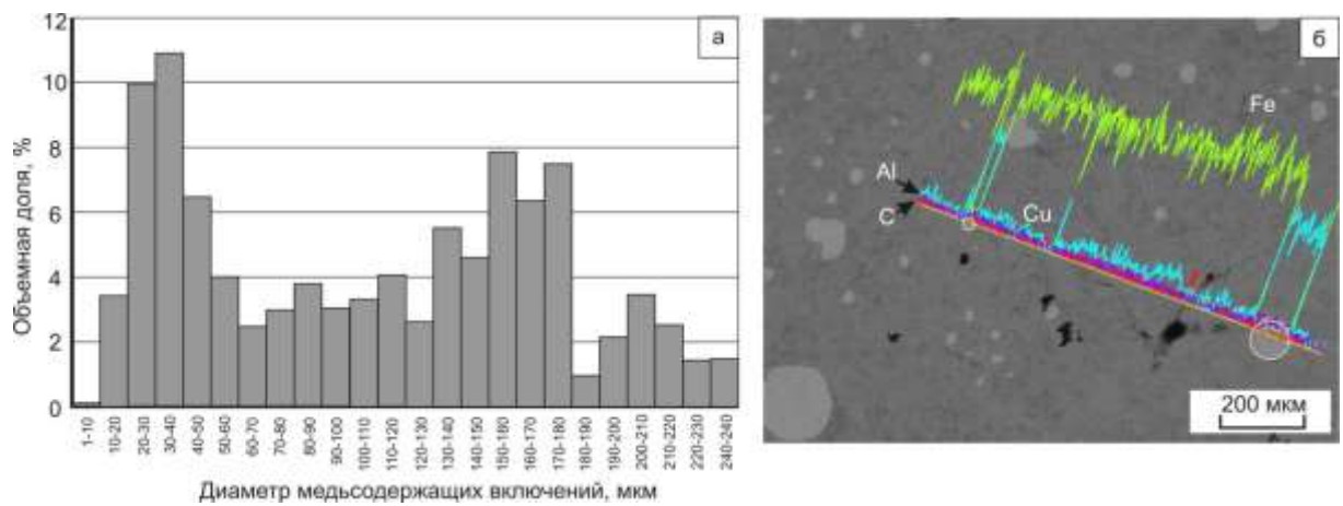
Рисунок 3.20 – Распределение по размерам медистых включений 1 и 2 типов (а) и распределение химических элементов вдоль линии, проходящей через включения разного размера в чугунах с 14,7 % Cu (б)
