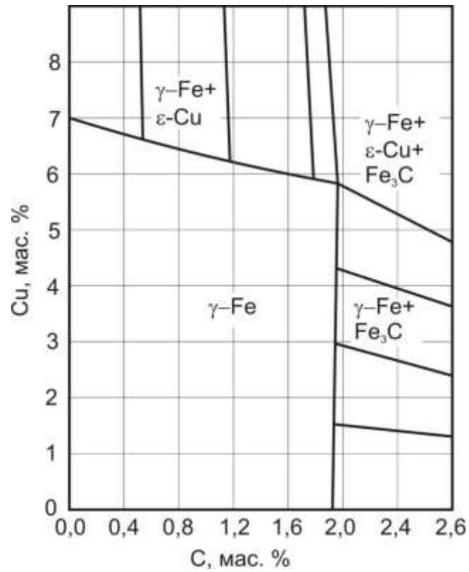
Рисунок 1.7 - Железный угол изотермического разреза диаграммы Fe\text{-Cu-C} при 1100 °C [132].
