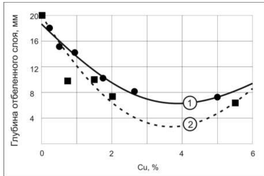
Рисунок 1.10 – Влияние содержания меди в сером чугуне на глубину отбеленного слоя, 1 – данные работы [93], 2 – данные работы [35]
