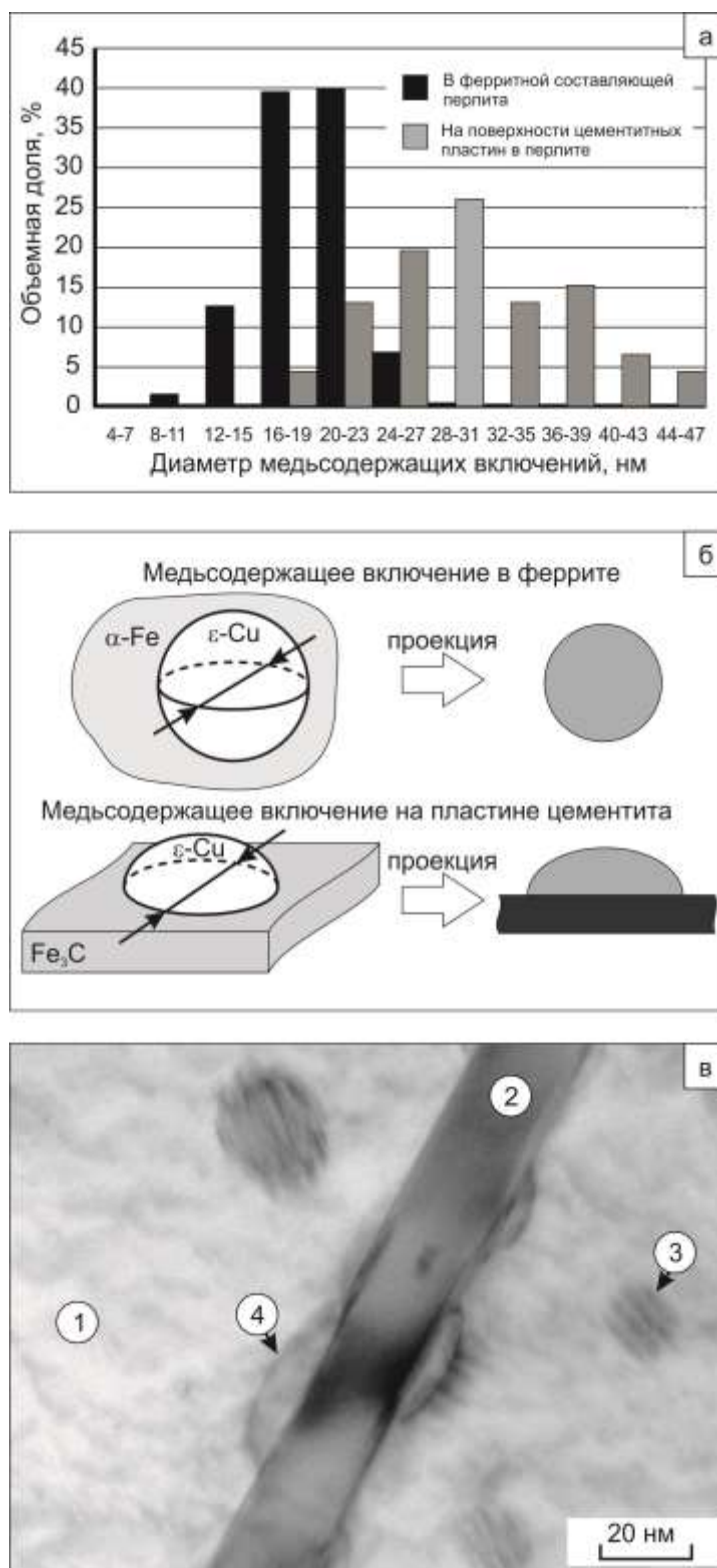
Рисунок 3.18 – Особенности выделения \epsilon\text{-Cu} в перлите: а - распределение частиц \epsilon\text{-Cu} по размерам; б – виды частиц \epsilon\text{-Cu} в перлите; в – ПЭМ перлита, содержащего частицы \epsilon\text{-Cu}
