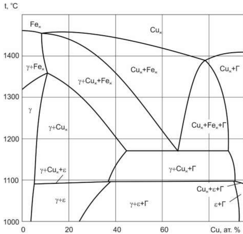
Рисунок 1.6 – Разрез диаграммы Fe-Cu-C при 5 мас. % углерода [130]
