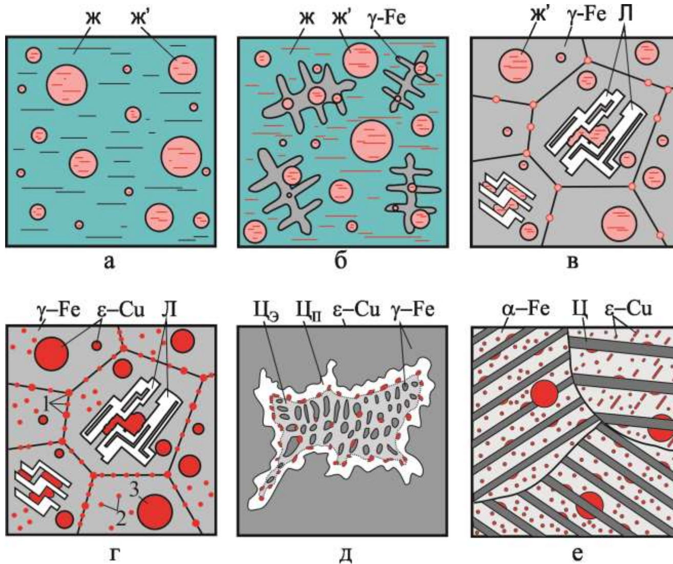
Рисунок 3.12 - Особенности выделения обогащенной медью фазы в чугунах, содержащем 2,9 % C и 14,7 % Cu. Л – ледебурит, Ц Э и Ц II – кристаллы эвтектического и вторичного цементита
