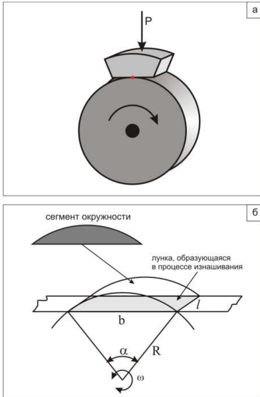
Рисунок 2.5 – Схема испытания диск – плоскость (а) и схематичное изображение лунки изнашивания (б)
