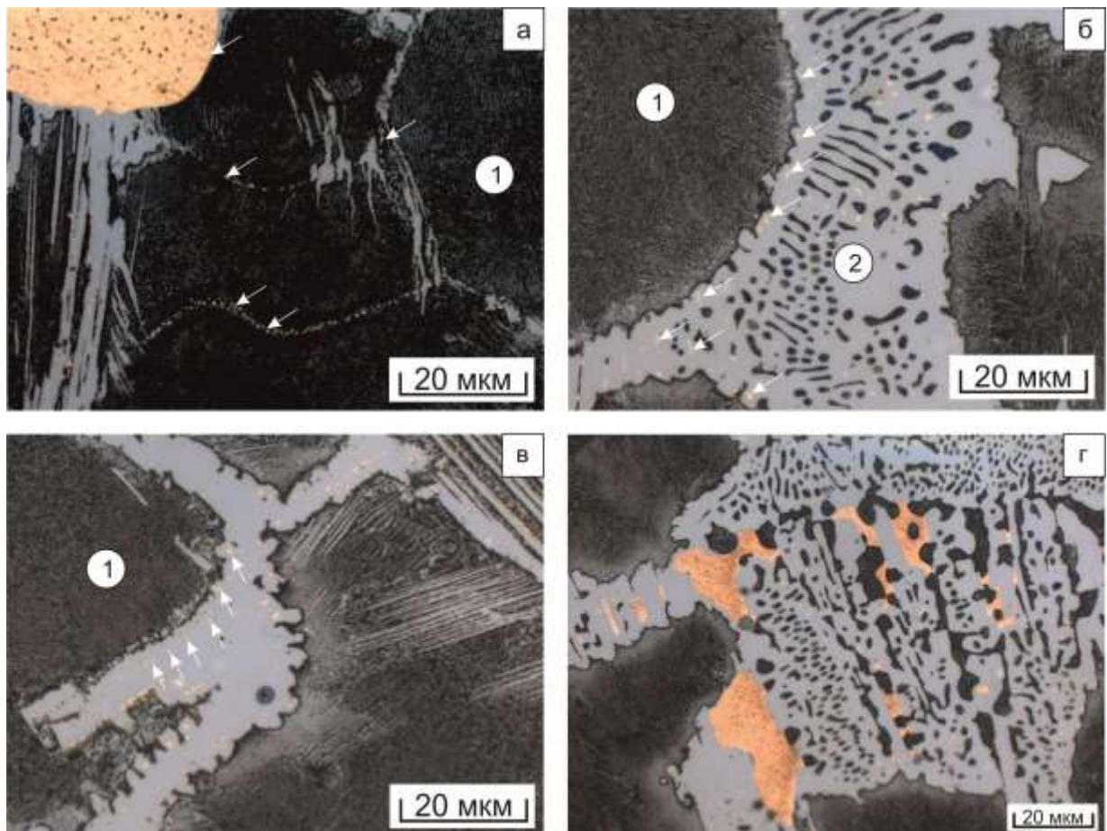
Рисунок 3.19 – Структура чугуна, содержащего 14,7 % Cu (1 – перлит, 2 – ледебурит). Стрелками показаны медистые включения
