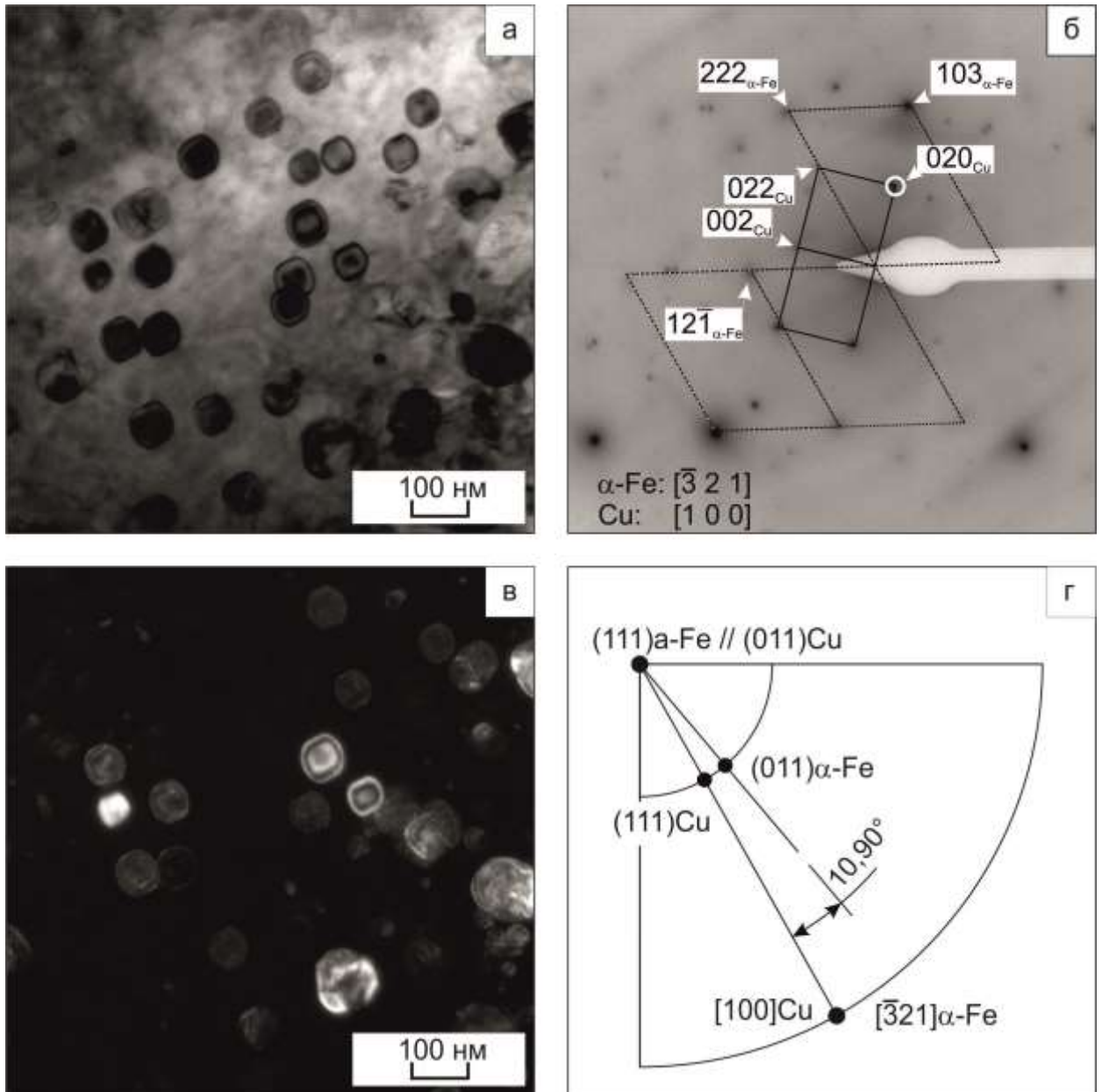
Рисунок 3.17 – Просвечивающая электронная микроскопия чугуна, содержащего мелкодисперсные включения фазы \epsilon -Cu
