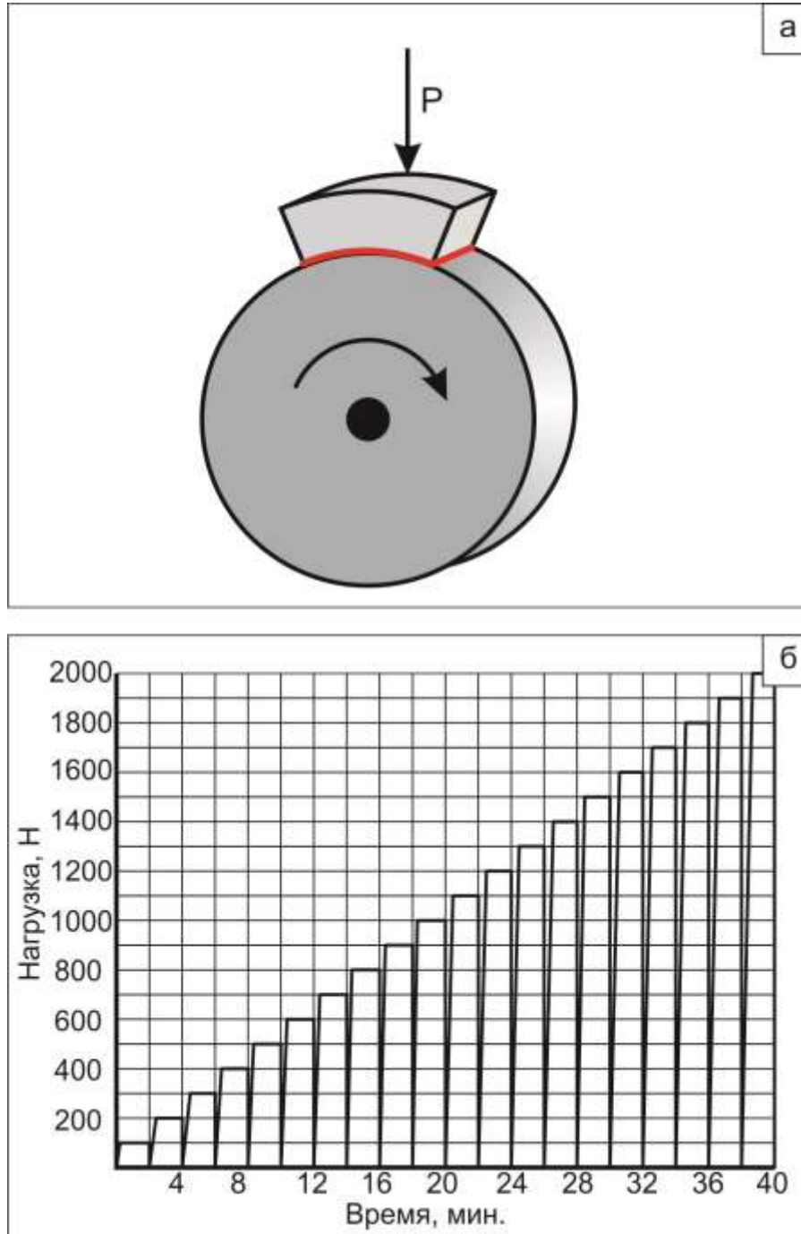
Рисунок 2.4 – Схема триботехнических испытаний "диск – колодка" (а) и график нагружения образцов при проведении экспериментов (б)
