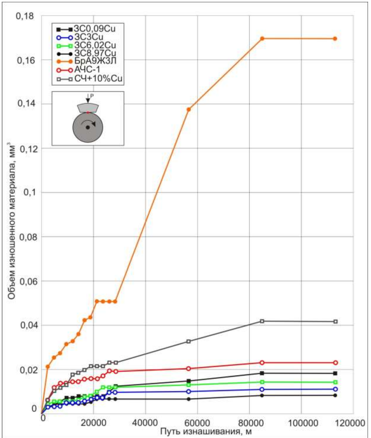
Рисунок 4.13 – Зависимости значений объема изношенного материала от пути трения по схеме врезавшегося индентора для образцов из заэвтектоидных сталей с различным содержанием меди, а также из бронзы БрА9Ж3Л и антифрикционного чугуна АЧС-1
