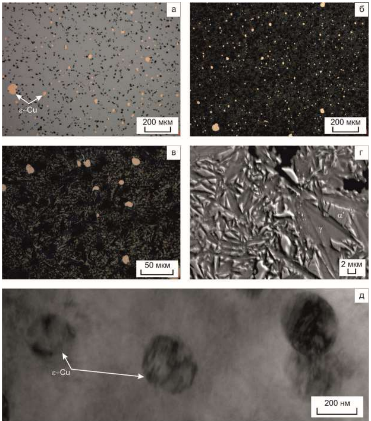
Рисунок 3.27 – Структура чугуна, легированного медью, после закалки от 1000 °C
