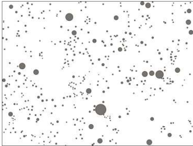
Рисунок 3.18 – Распределение частиц \epsilon -Cu 1 и 2 типов
