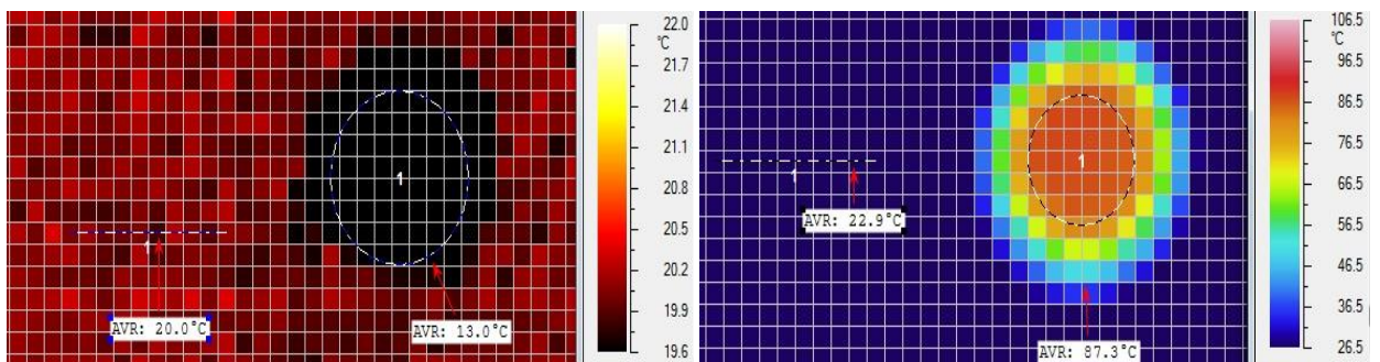
Рисунок 3.3 – Характерные тепловизионные изображения торца оптического волокна при температуре источника теплового излучения 271,5 К и 400 К соответственно, полученные в длинноволновом диапазоне с помощью тепловизора NEC 7102WV.
