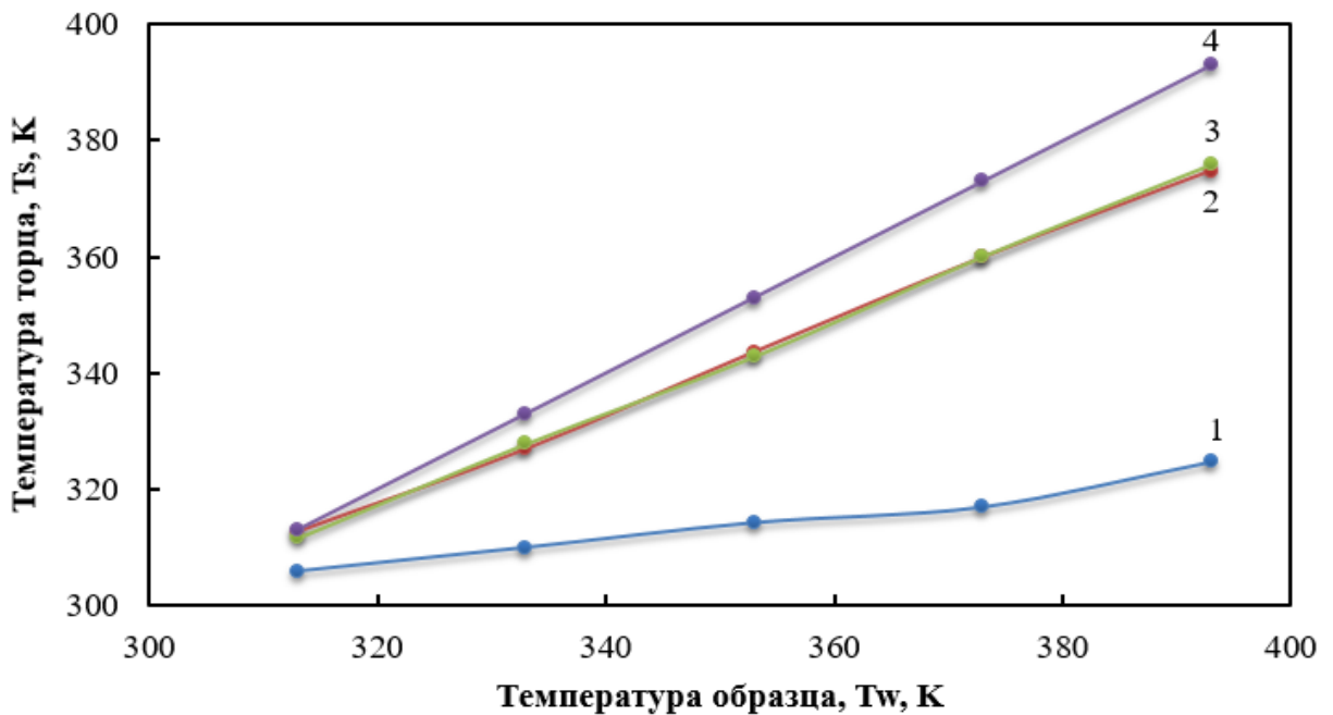
Рисунок 3.7 – Температура на выходном торце световода T_s при различной температуре поверхности образца T_w : 1 – при d = 0,5 мм, 2 – при d = 1,12 мм, 3 – при d = 1,75 мм, 4 – при отсутствии потерь.
