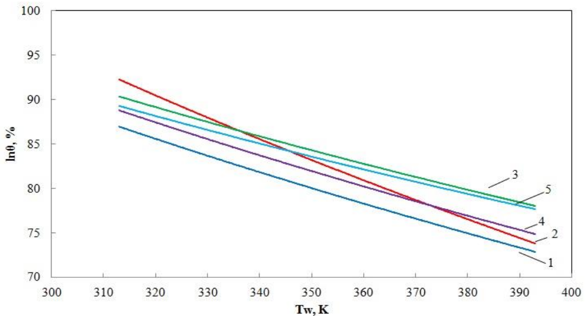
Рисунок 3.11 – Доля пропускания теплового излучения \theta через световод состава AgCl_{0,75}Br_{0,25} диаметром d = 1,12 мм при различной температуре поверхности образца T_w : 1 – без изоляции, 2 – алюминиевая фольга, 3 – фторопласт, 4 – пенопласт, 5 – изолон.
