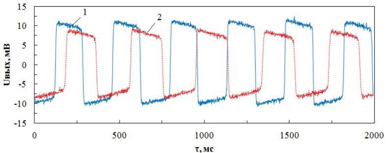
Рисунок 3.24 – Временные характеристики выходного напряжения U_{\text{вых}} для канала со световодами разных составов: 1 – \text{AgCl}_{0,25}\text{Br}_{0,75} и; 2 – \text{Ag}_{0,95}\text{Tl}_{0,05}\text{Br}_{0,95}\text{I}_{0,05} .
