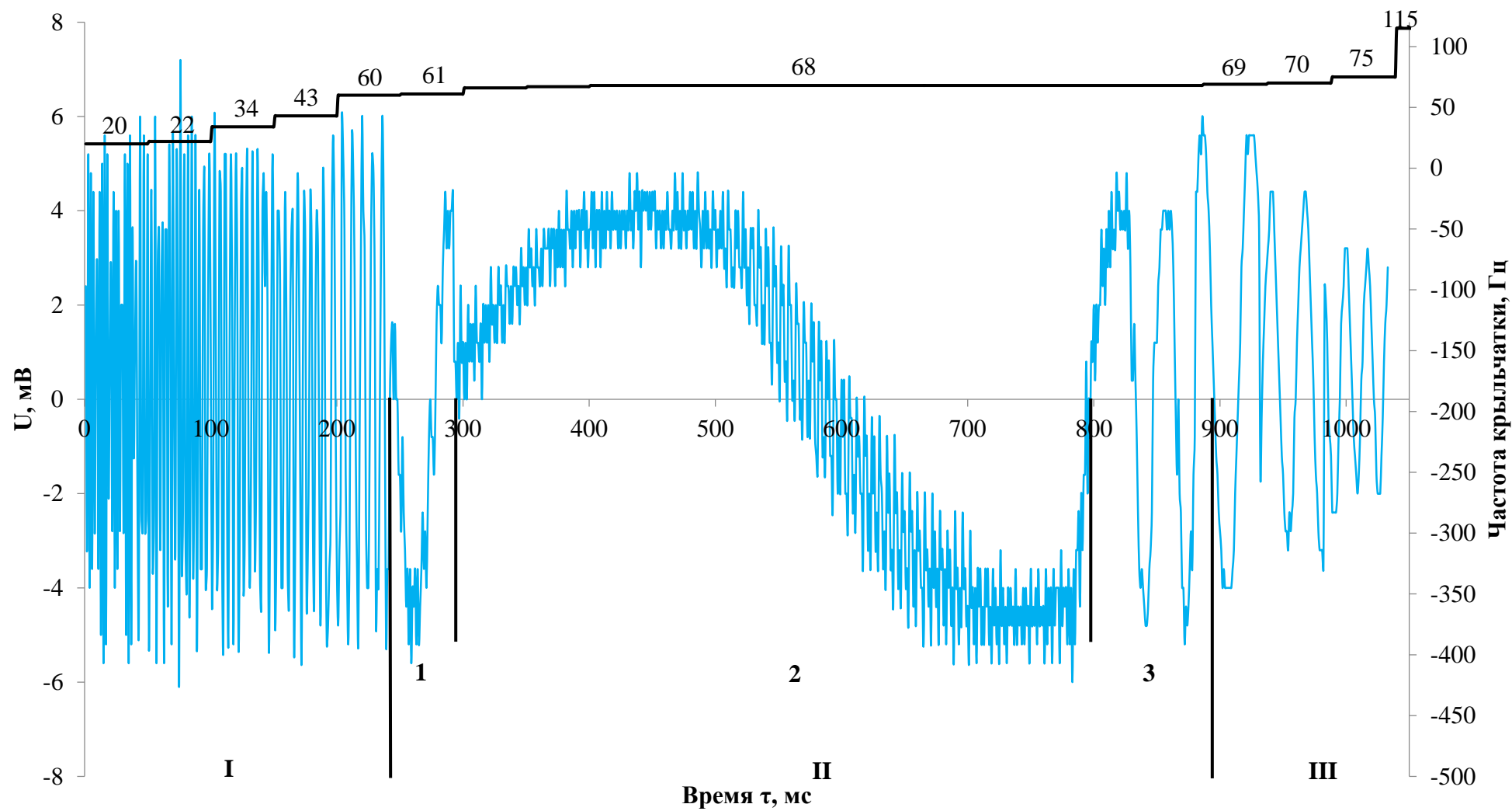
Рисунок 3.16 – График зависимости колебаний выходного напряжения предусилителя U во времени \tau от частоты крыльчатки.
