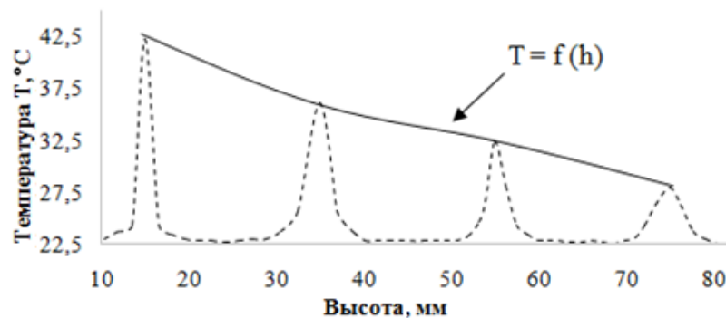
Рисунок 4.3 – График распределения температуры по высоте рабочей лопатки ГТУ.
