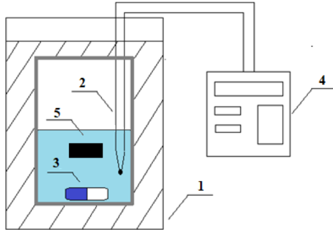
Рисунок 3.32 – Схематическое изображение экспериментальной установки для определения удельной теплоемкости световодов: 1 – теплоизоляционная оболочка со стаканом; 2 – термопара; 3 – магнитная мешалка; 4 – измеритель ОВЕН ТРМ-151; 5 – образец.
