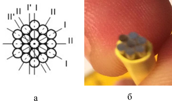
Рисунок 3.12 – Гексагональный вертикальный тип укладки волокон (а) и – фотография принимающего торца волоконно-оптической сборки (б).
