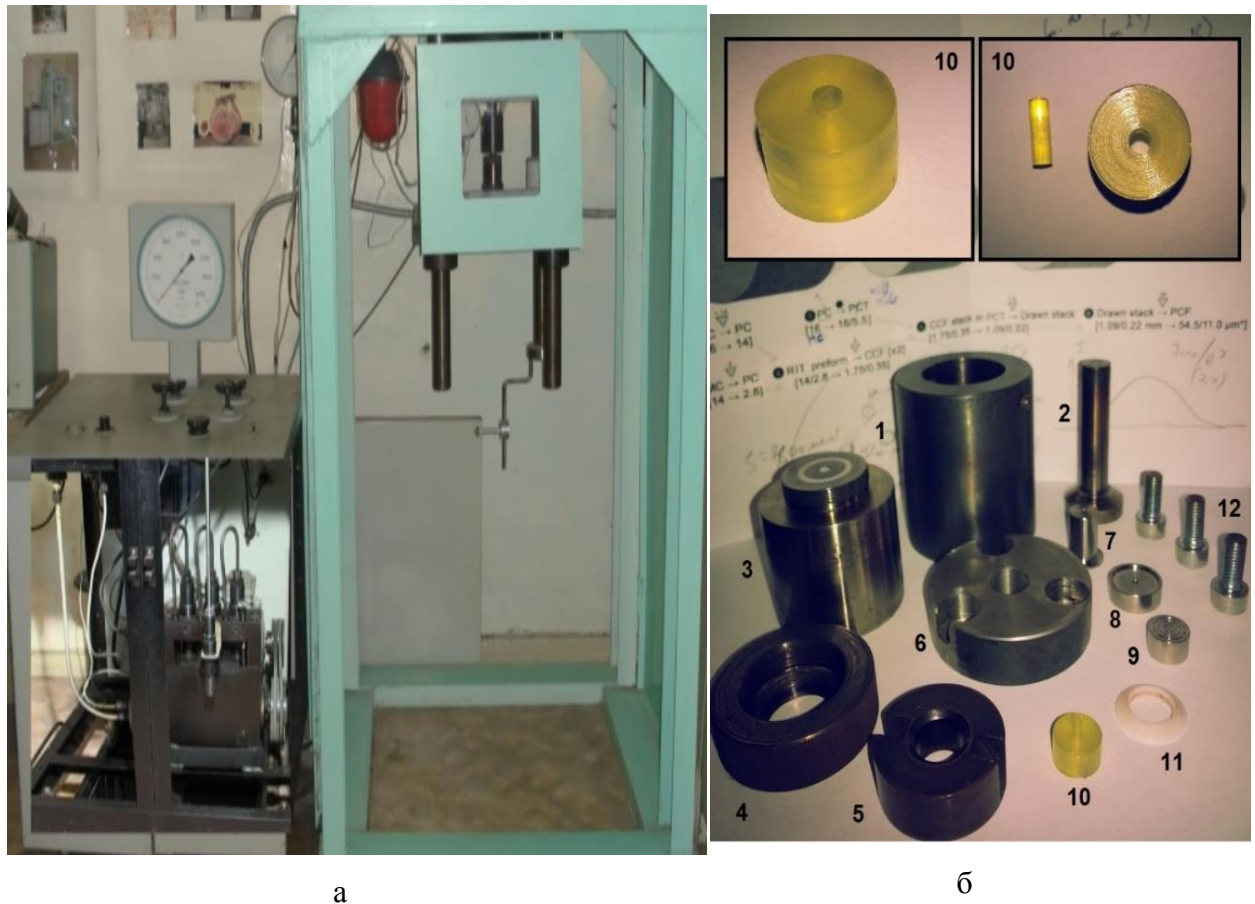
Рисунок 2.10 – Общий вид прессы ПОИ-500 (а) и оснастки для прессования (б): 1 – контейнер; 2 – давящий плунжер; 3 – основание плунжера; 4 – накидная гайка на плунжер; 5 – направляющая плунжера; 6 – крепеж; 7 – экструзионный плунжер; 8 – фильера; 9 – заглушка; 10 – заготовка-преформа; 11 – уплотнительное кольцо; 12 – болты для соединения контейнера и крепежа.
