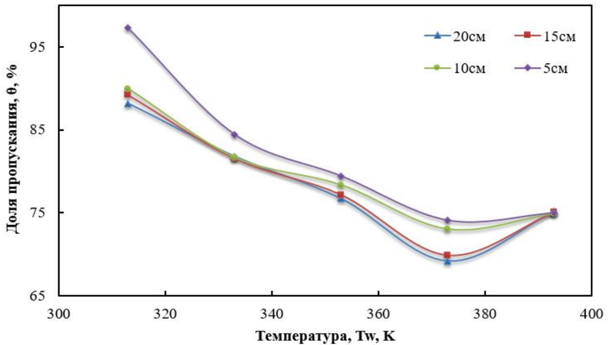
Рисунок 3.8 – Доля пропускания теплового излучения \theta через световод состава \text{AgCl}_{0,75}\text{Br}_{0,25} диаметром d = 1,75 мм при различной температуре поверхности образца T_w для различных длин исследуемого ИК световода.
