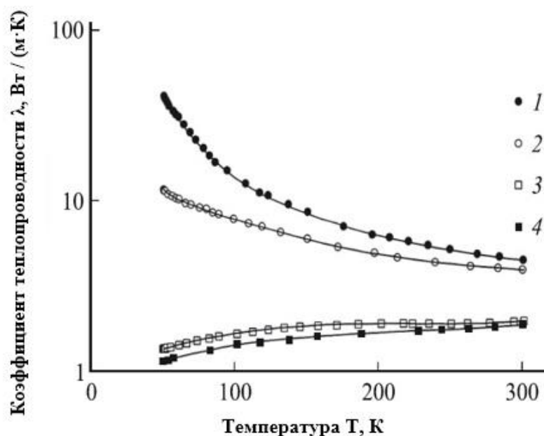
Рисунок 1.4 – Температурная зависимость теплопроводности монокристаллов CdF 2 легированных: 1 – CaF 2 , 2 – Ca 0.97 N 0.03 F 2.03 , 3 – Ca 0.85 Ho 0.15 F 2.15 , 4 – Cd 0.90 Er 0.10 F 2.10 [9].
