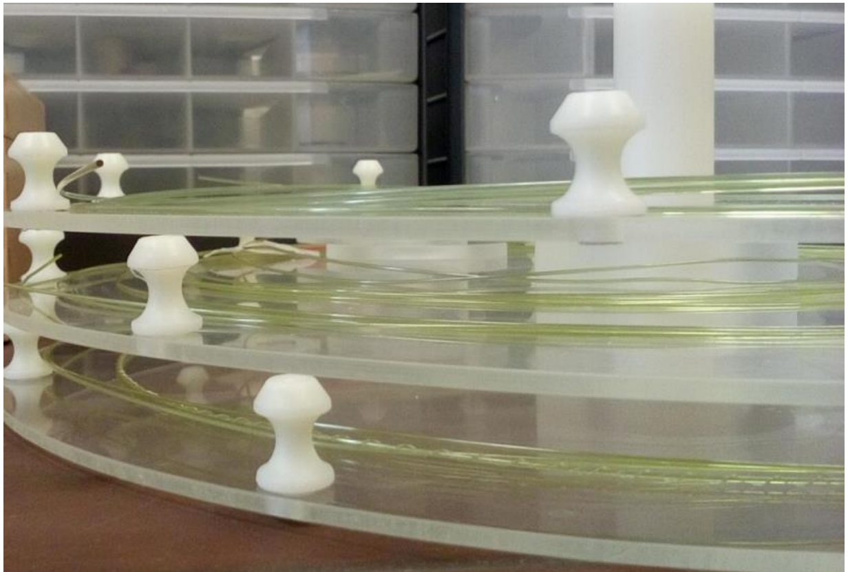
Рисунок 2.12 – Инфракрасные кристаллические световоды, изготовленные методом экструзии.
