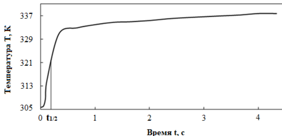
Рисунок 3.27 – График зависимости температуры T задней поверхности от времени t для пластины состава \text{AgCl}_{0,75}\text{Br}_{0,25} .
